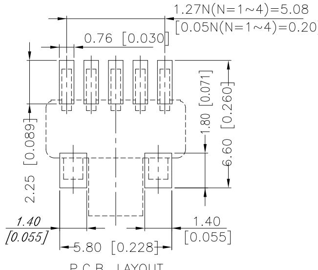
P.C.B. LAYOUT
